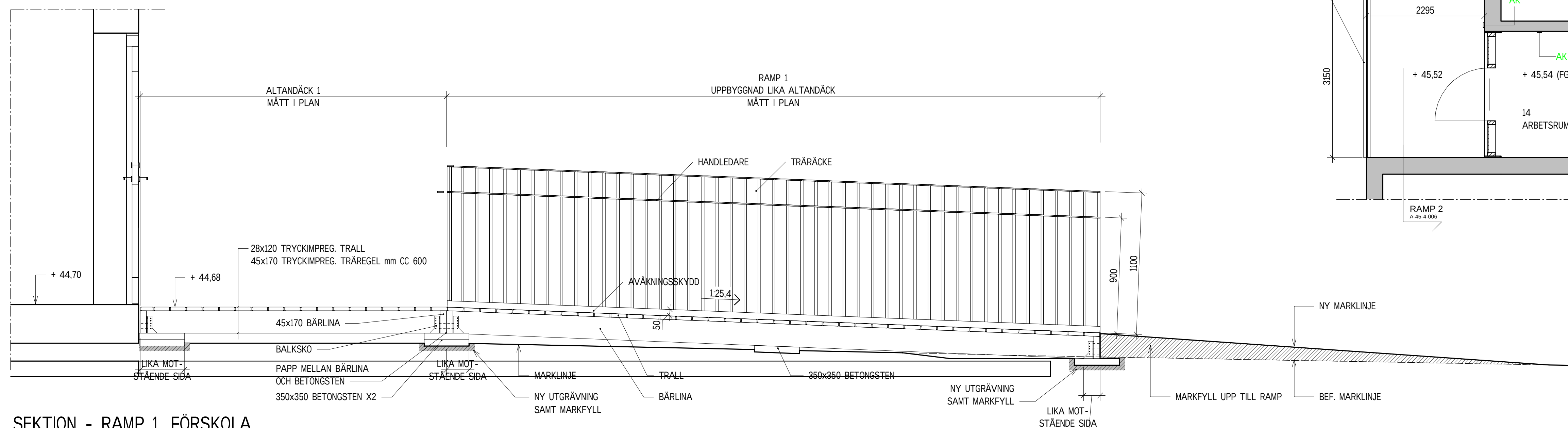
SEKTION - RAMP 1, FÖRSKOLA 1 : 20
