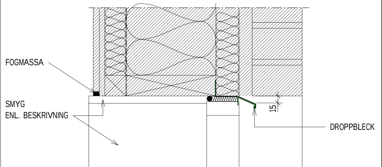
VD16 PRINCIPDETALJ 1:5 METALLPARTI
