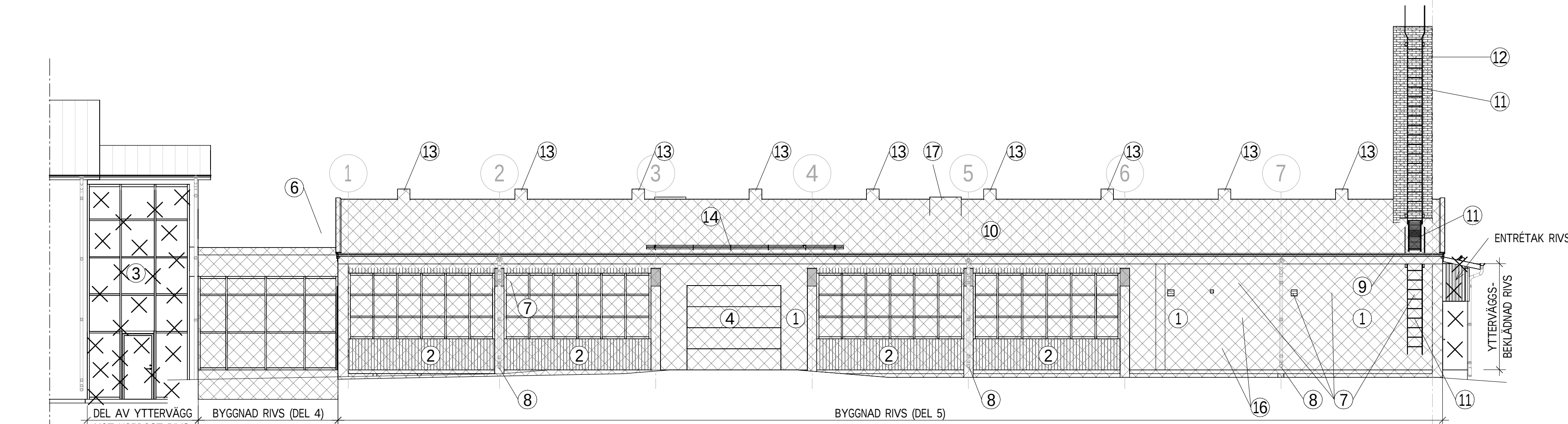
FASAD MOT NORDÖST - RIVNING
