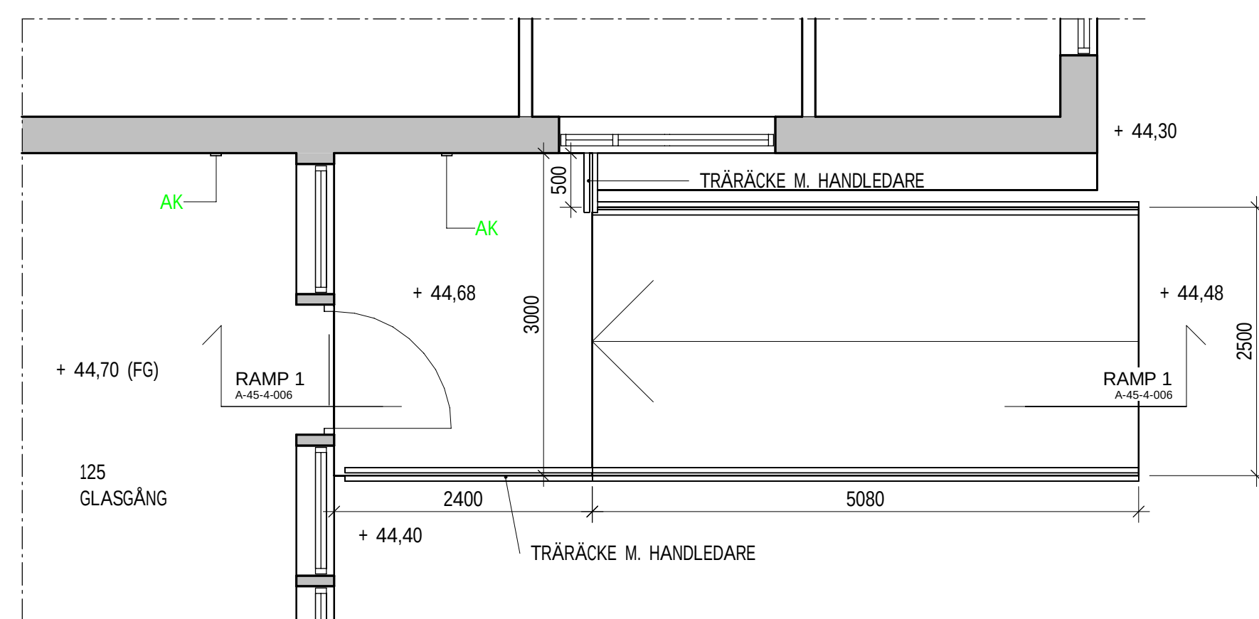
PLAN 1 - RAMP FÖRSKOLA 1 : 50
