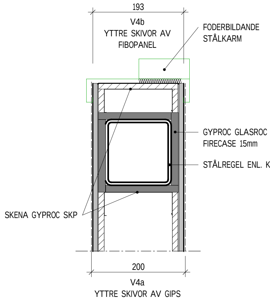
IK2 - STÅLPELARE I INNERVÄGG 1 : 5
