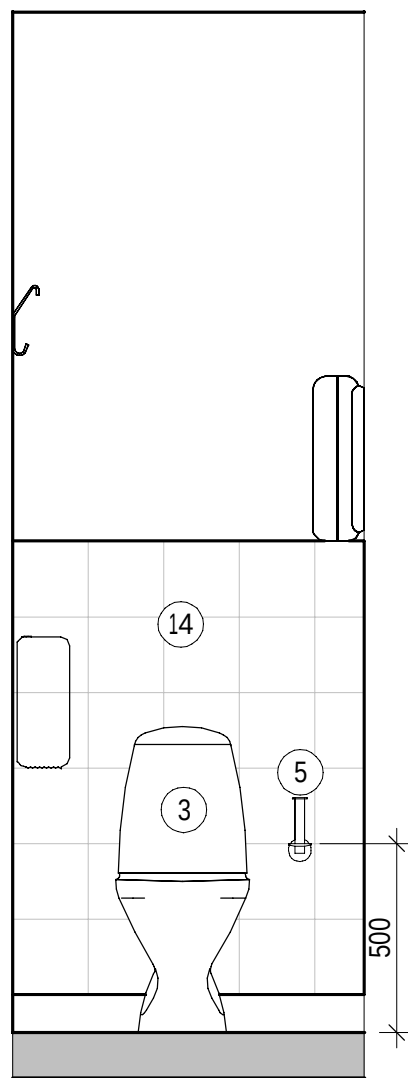
ELEVATION WC 1018 - A 1 : 20
