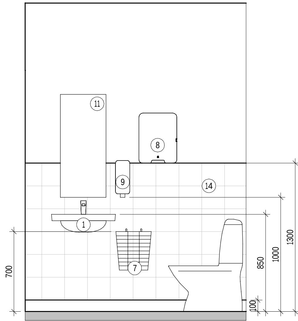
ELEVATION WC 1020 - C 1 : 20
