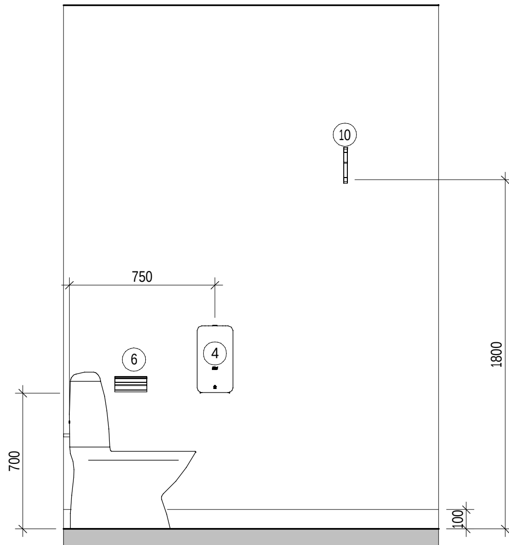
ELEVATION WC 1020 - A 1 : 20
