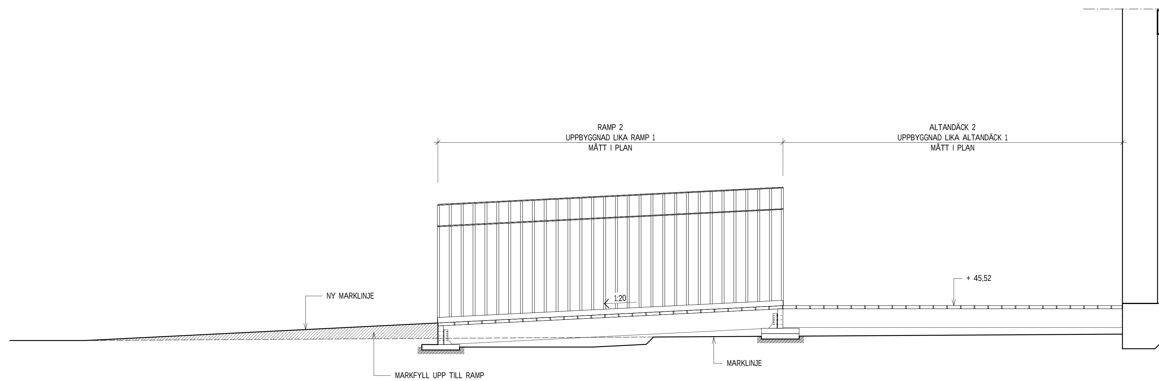
SEKTION - RAMP 2, FRITIDS 1 : 20
