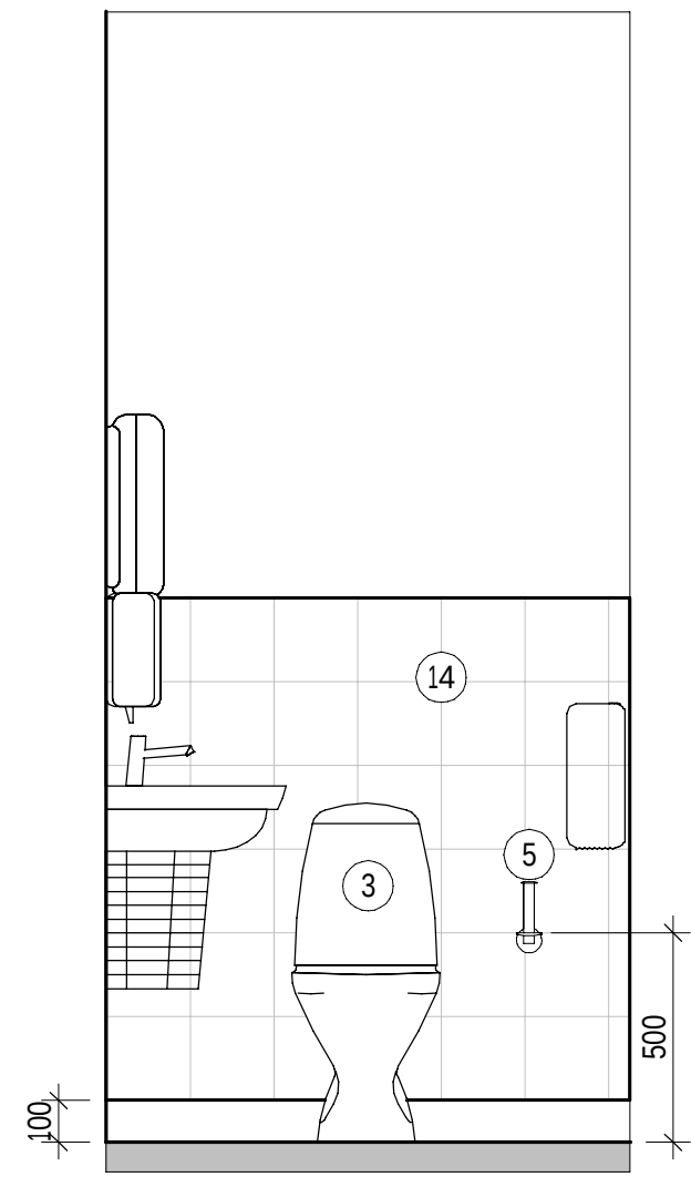
ELEVATION WC 1020 - D 1 : 20
