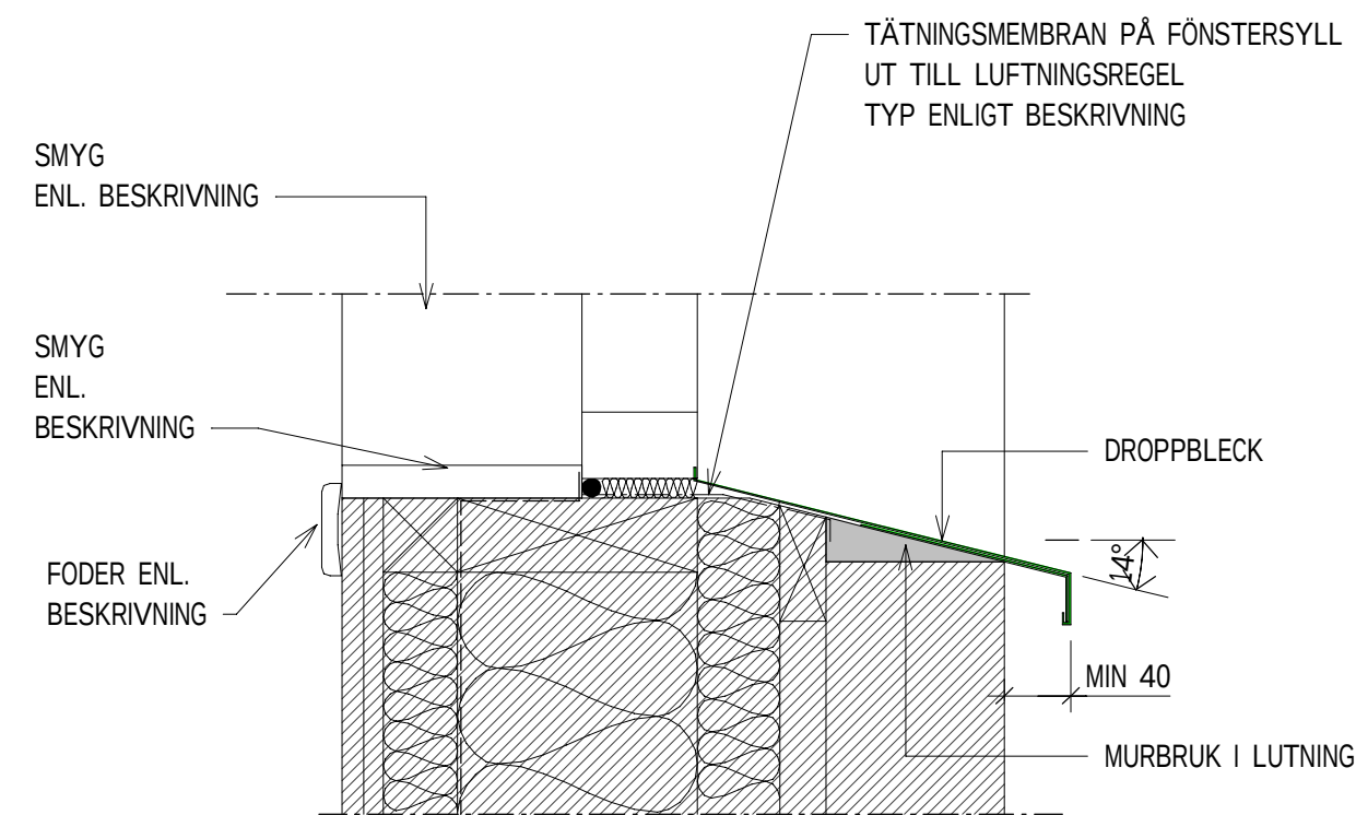
VD18 PRINCIPDETALJ 1:5 FÖNSTER SOPRUM
