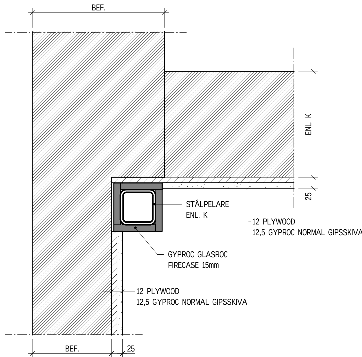
IK10 - STÅLPELARE VID BEF. VÄGGHÖRN 1 : 5
