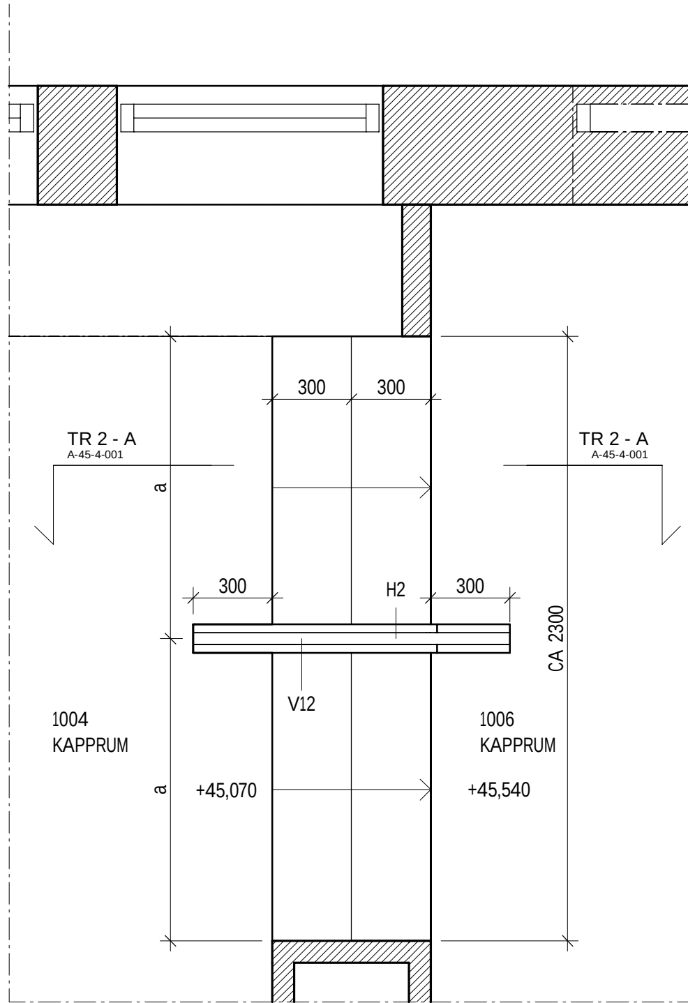
TRAPPA 2 - PLAN 1 : 20
