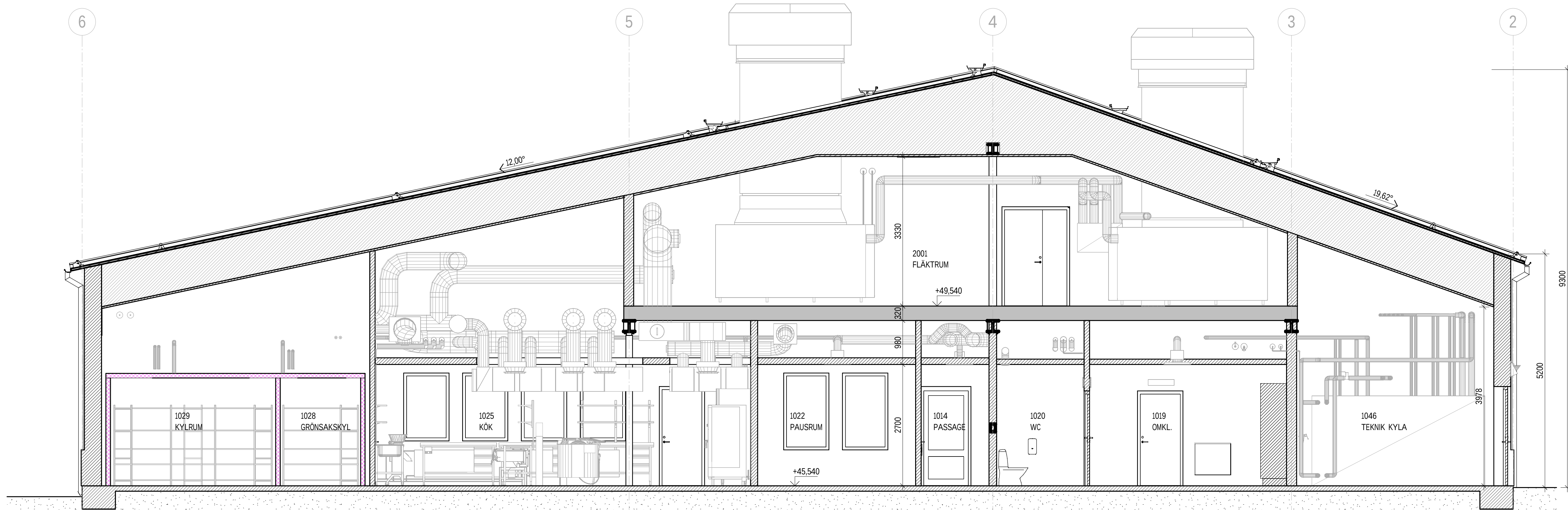
SEKTION A 1 : 50
