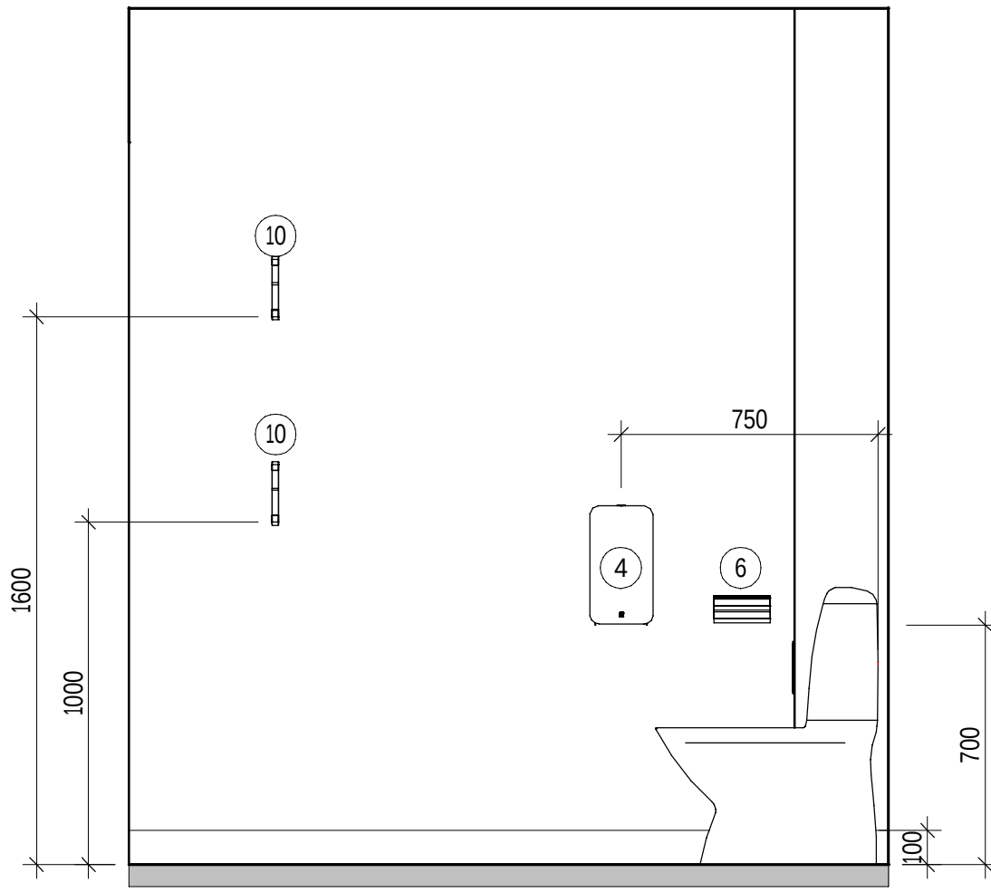
ELEVATION WC 1008 - D 1 : 20
