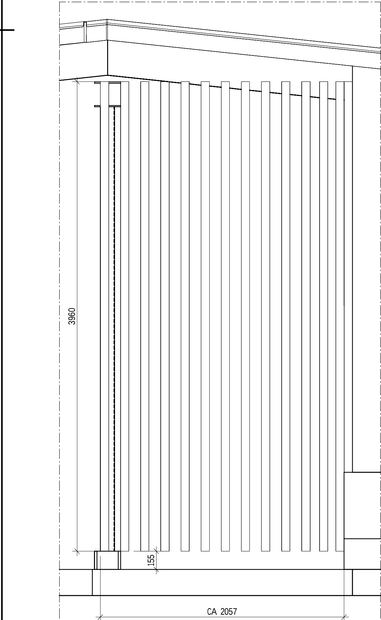
Elevation - SPALJÉ 2 1 : 20
