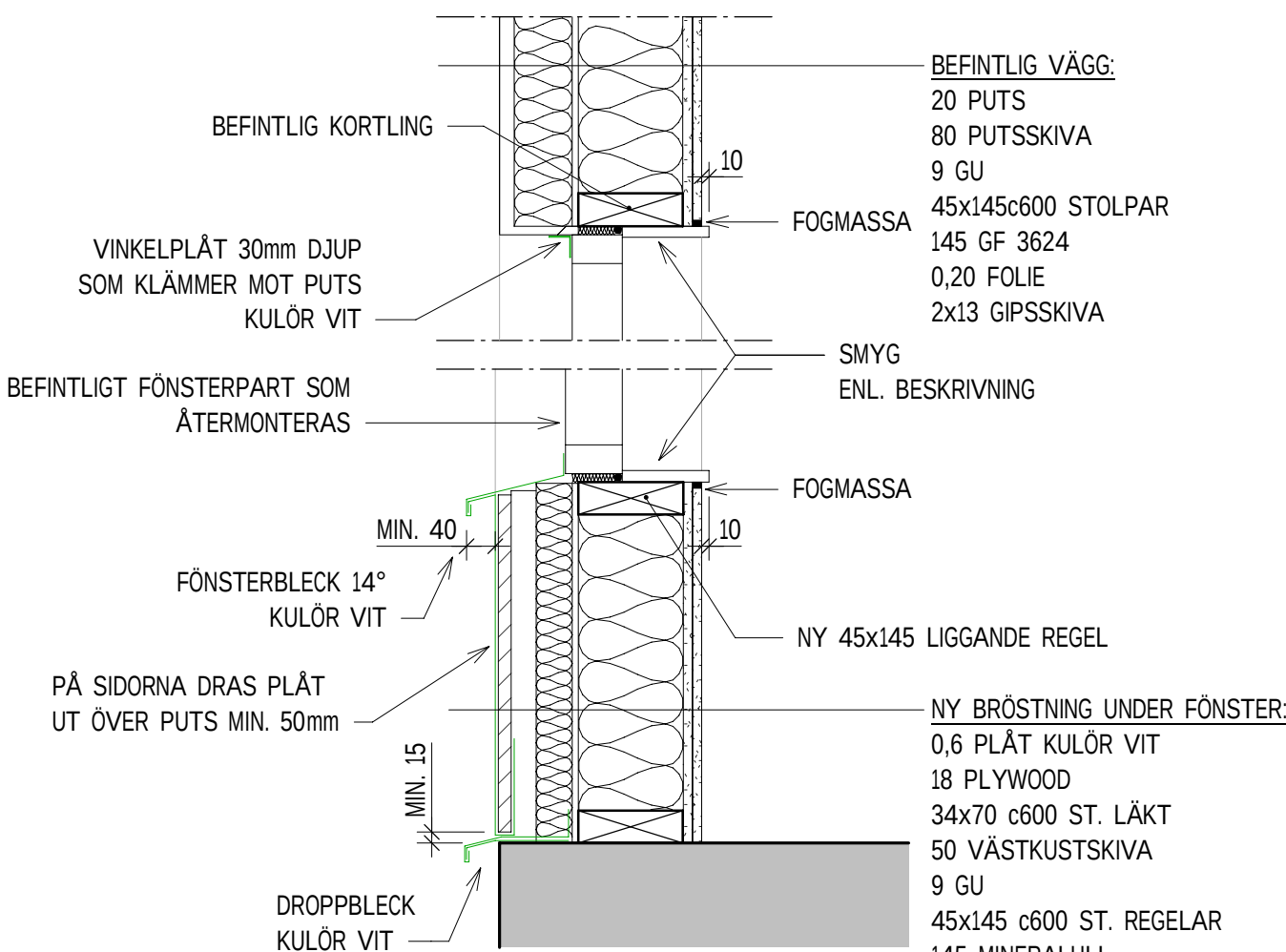
VD22 - IGENBYGGNAD FÖNSTER FRITIDS 1:10
