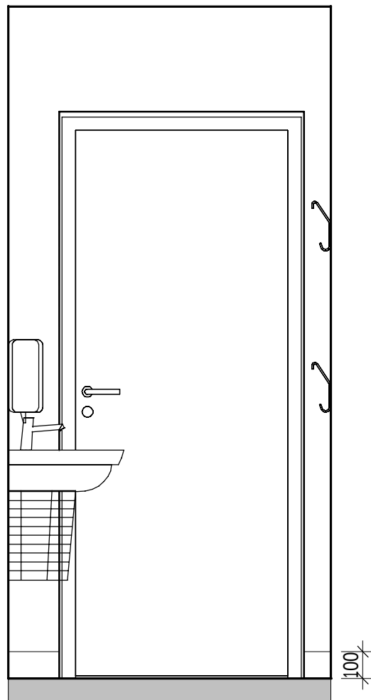
ELEVATION WC 1008 - C 1 : 20
