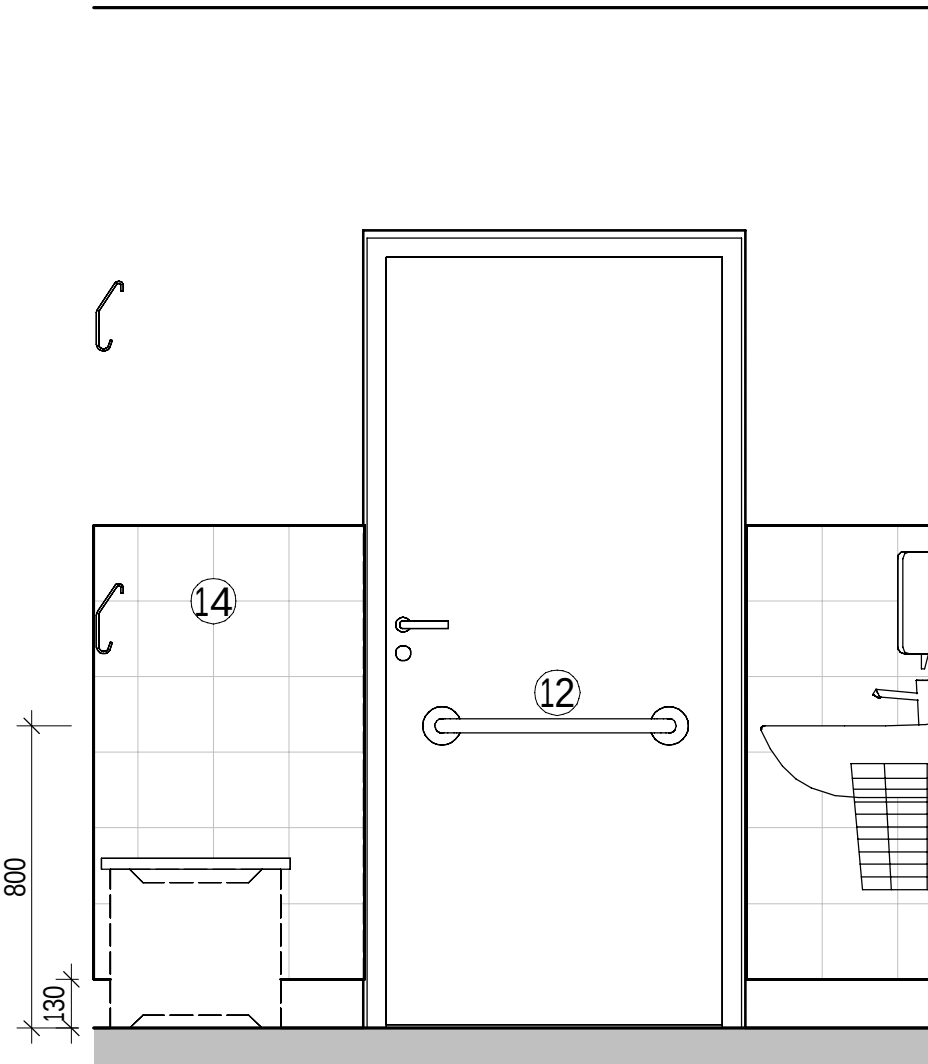
ELEVATION RWC/D 1016-C 1 : 20
