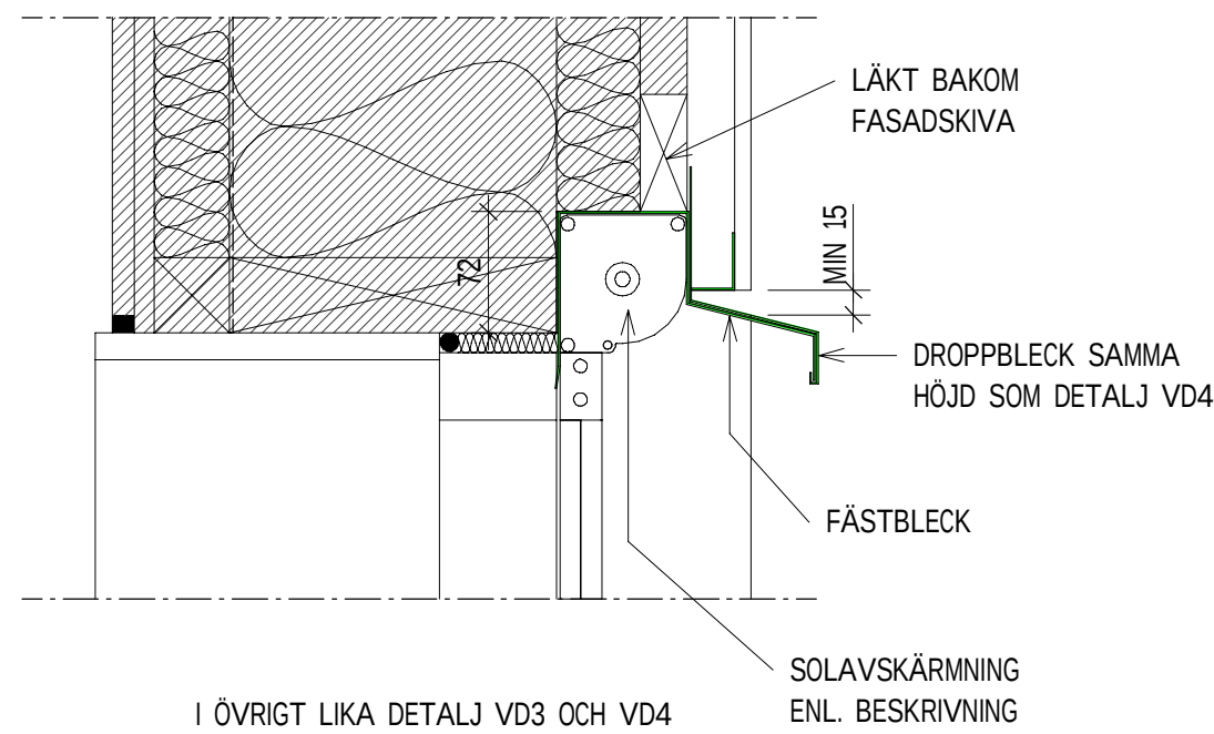
EV1 PRINCIP ELEVATION 1:10 RULLSKIFTS BALK - MED BYGEL
