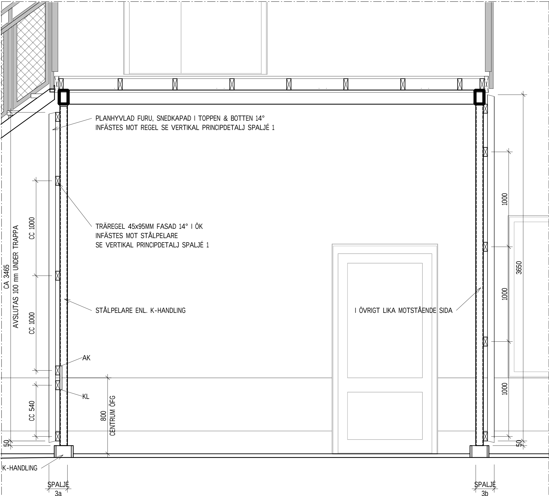
SPALJÉ 3 - SEKTION 1 : 20
