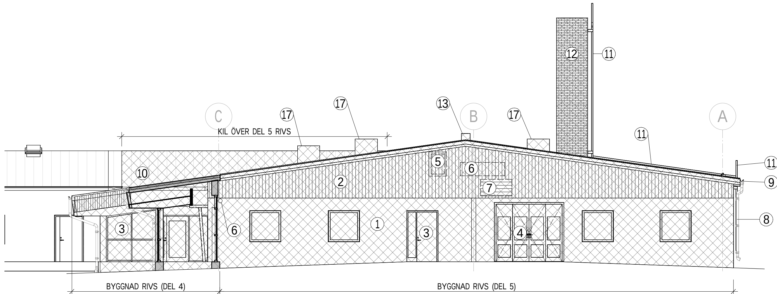
FASAD MOT SYDÖST - RIVNING
