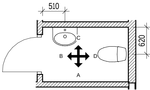
PLAN WC 1020 1 : 50
