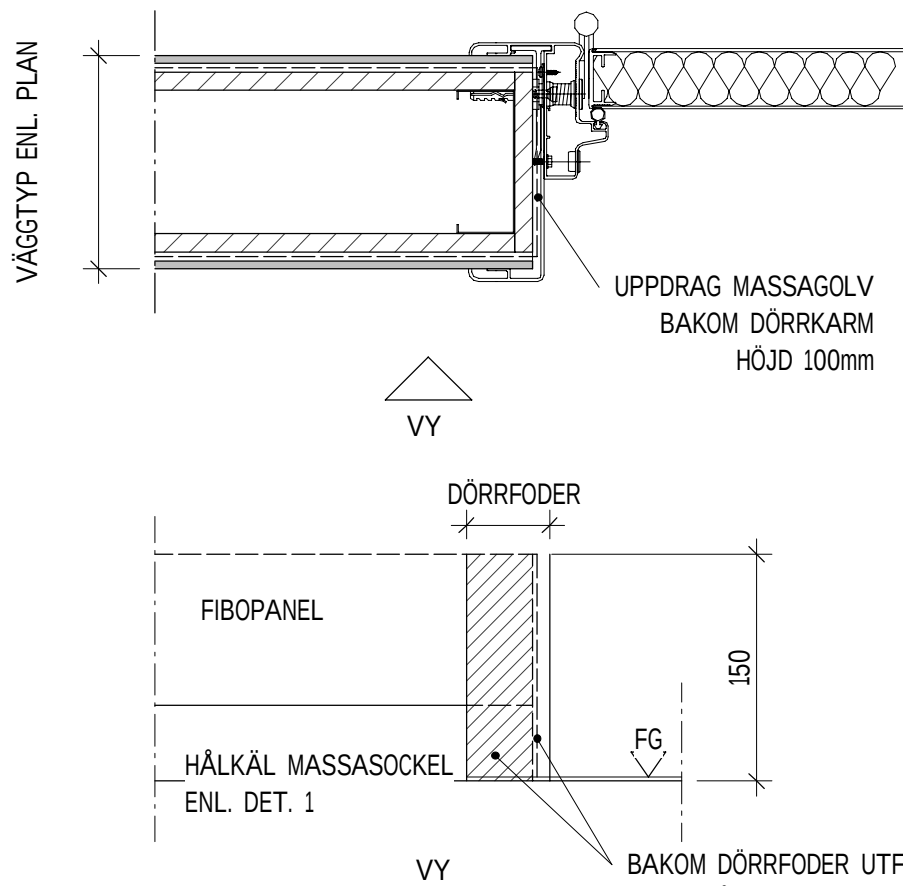
IVD01 - PRINCIPDETALJ MÖTE INNERVÄGG 1 : 5
