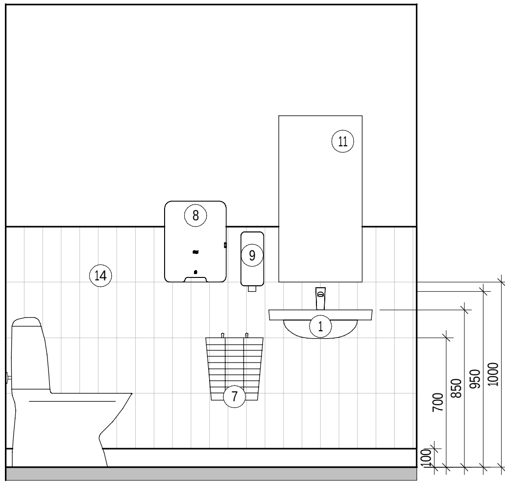
ELEVATION WC 1008 - B 1 : 20
