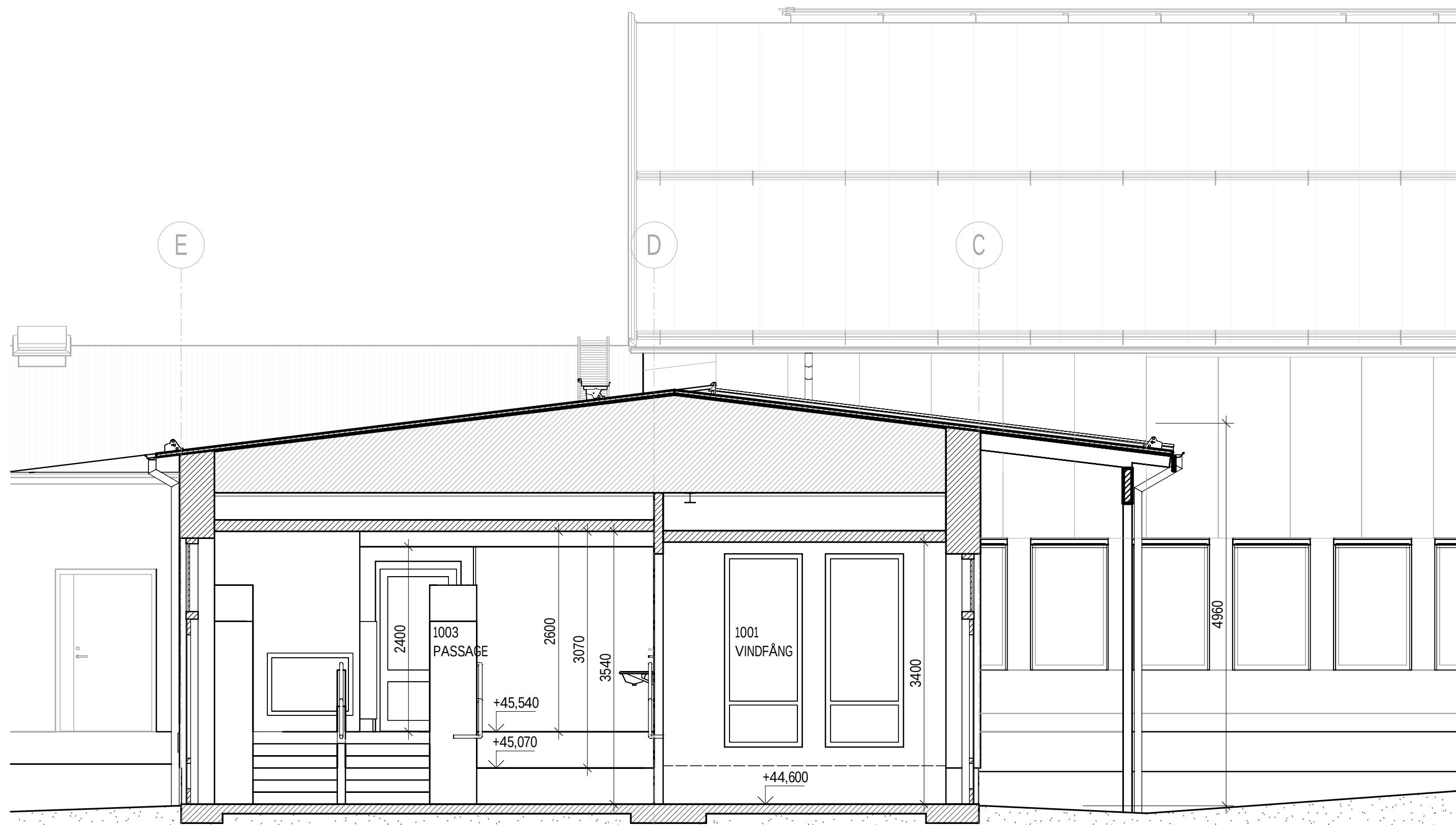
SEKTION A 1 : 50
