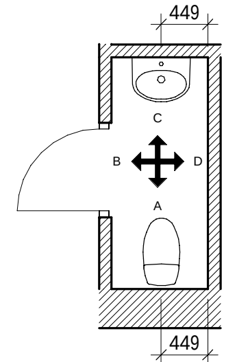
PLAN WC 1018 1 : 50
