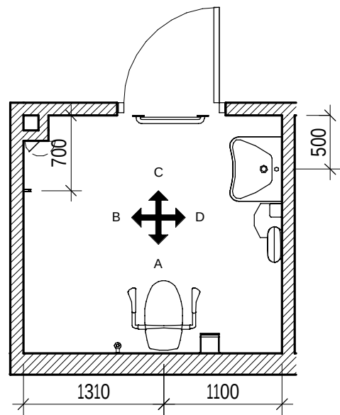
PLAN RWC 1007 1 : 50
