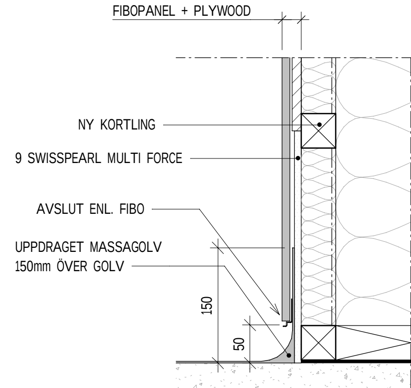
IVD11 - PRINCIPDETALJ MASSAGOLV MOT YTTERVÄGG 1 : 5
