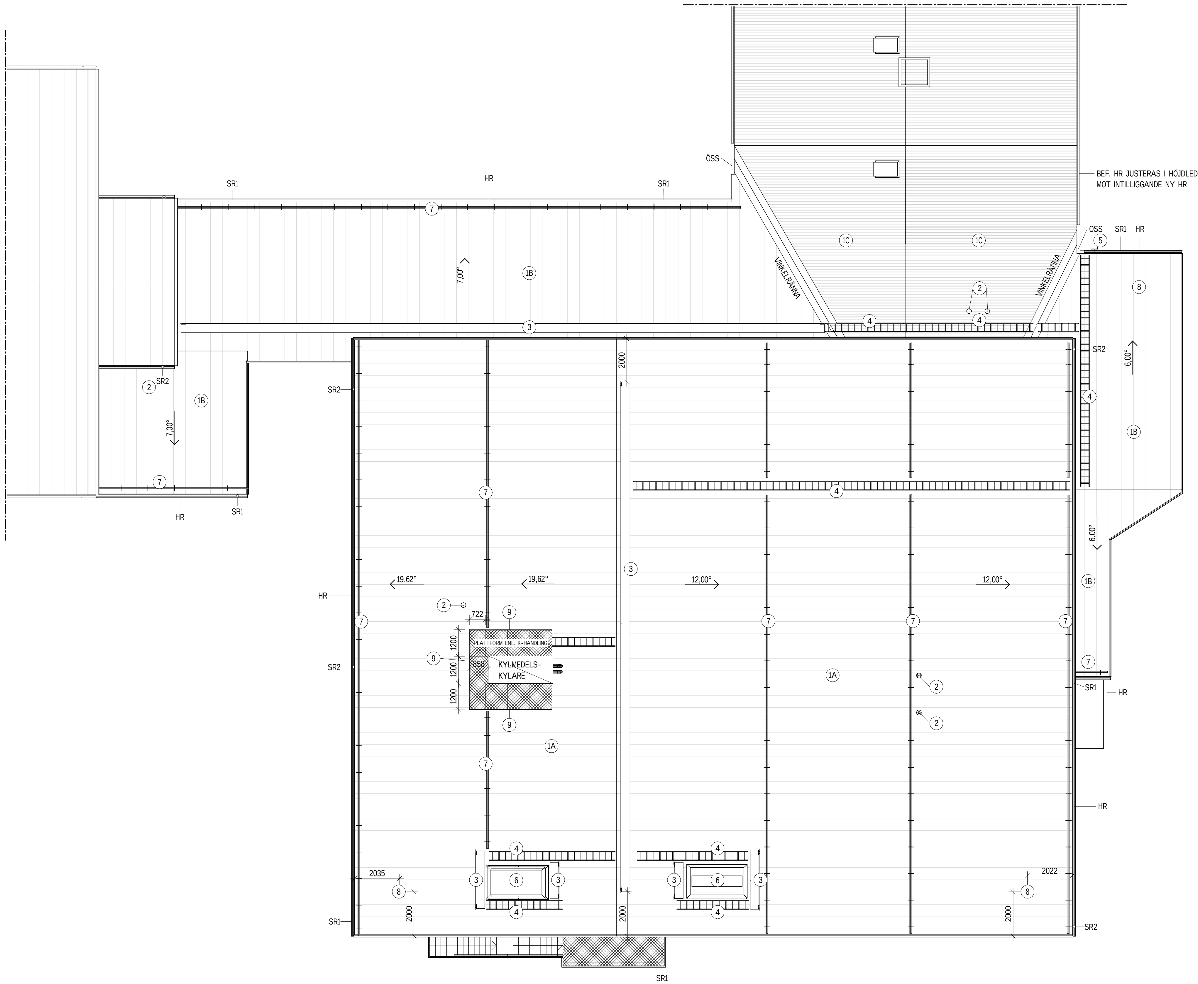
TAKPLAN 1 : 100
