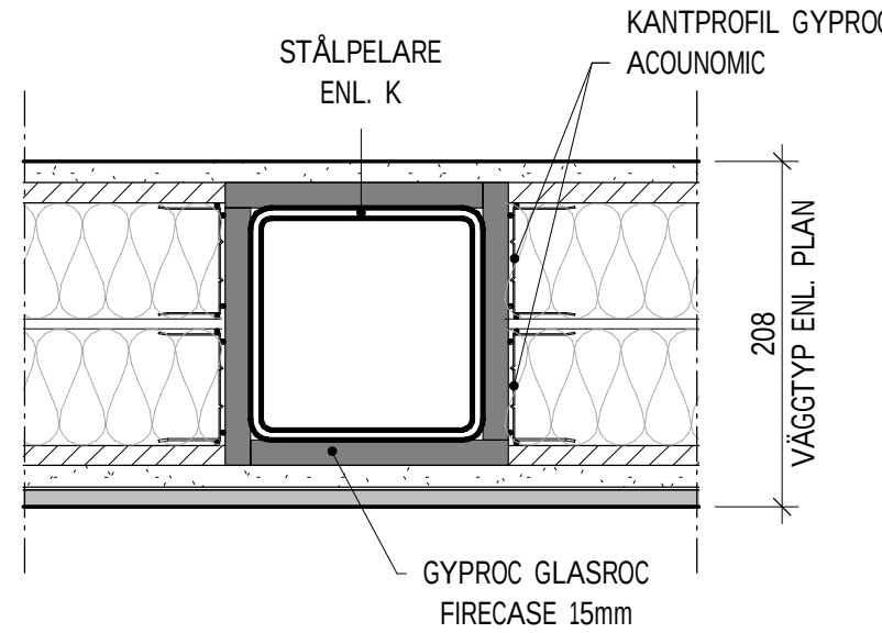
IK3 - STÅLPELARE I DUBBELREGLVÄGG 1 : 5
