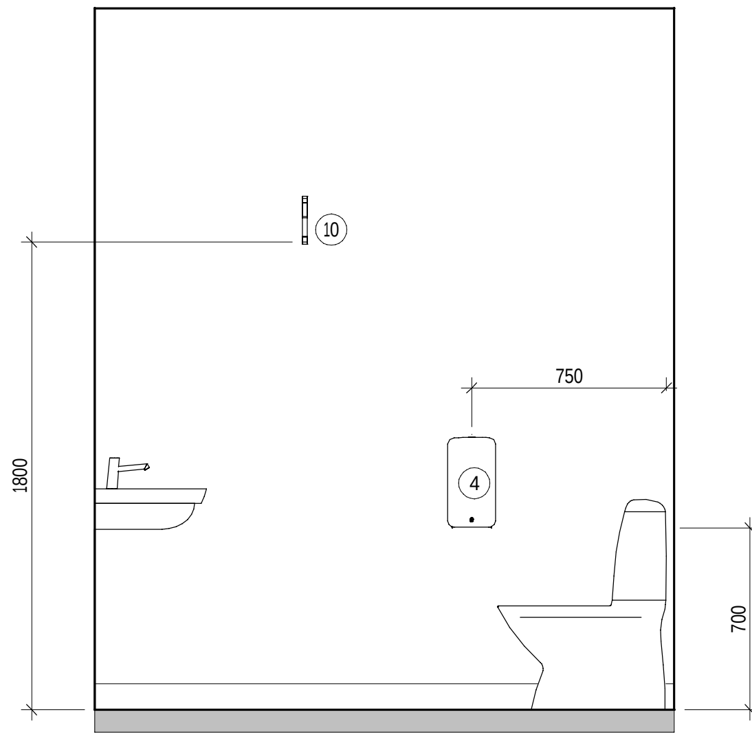
ELEVATION WC 1018 - D 1 : 20
