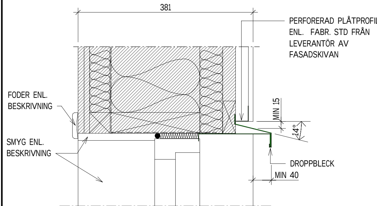
VD8 PRINCIPDETALJ 1:5 DÖRR FLÄKTRUM PLAN 2
