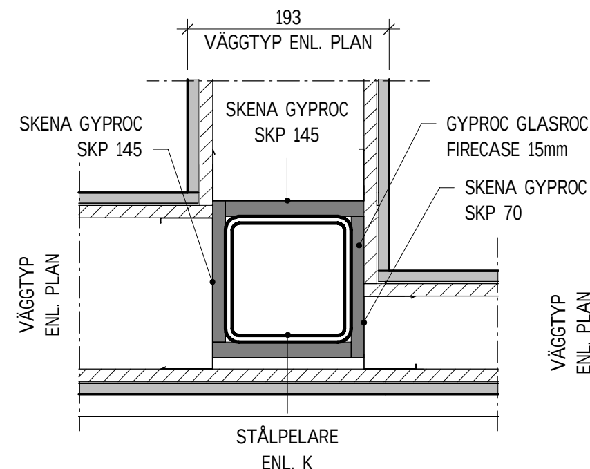
IK7 - STÅLPELARE I VÄGGKORSNING KÖK 1 : 5
