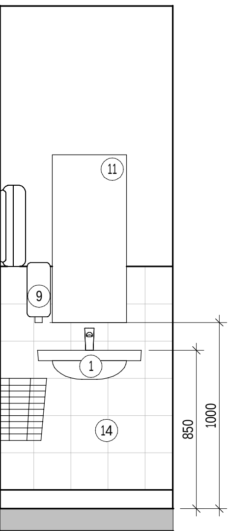
ELEVATION WC 1018 - C 1 : 20
