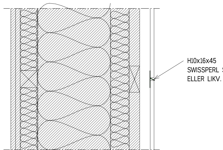
VD20 PRINCIPDETALJ 1:5 LIST MELLAN FASADSKIVOR
