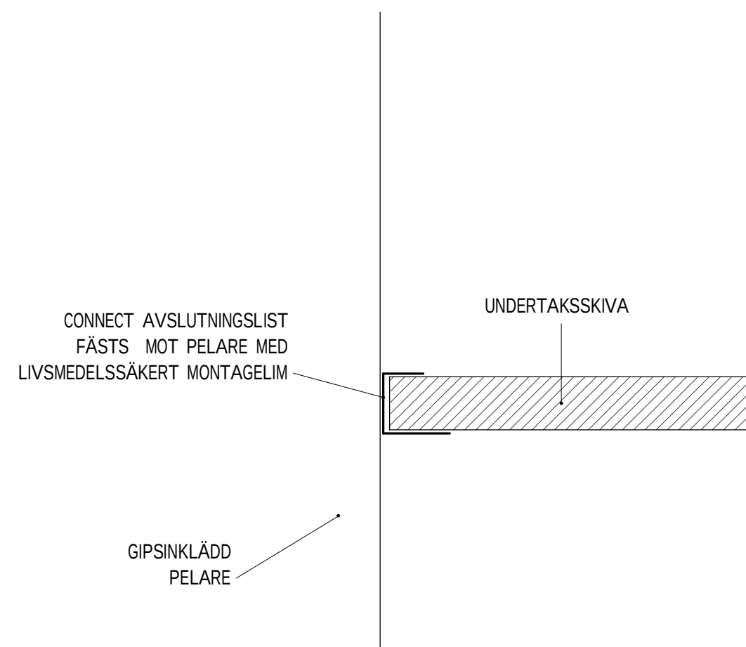
UTD06 - ANSLUTNING MOT PELARE 1 : 2
