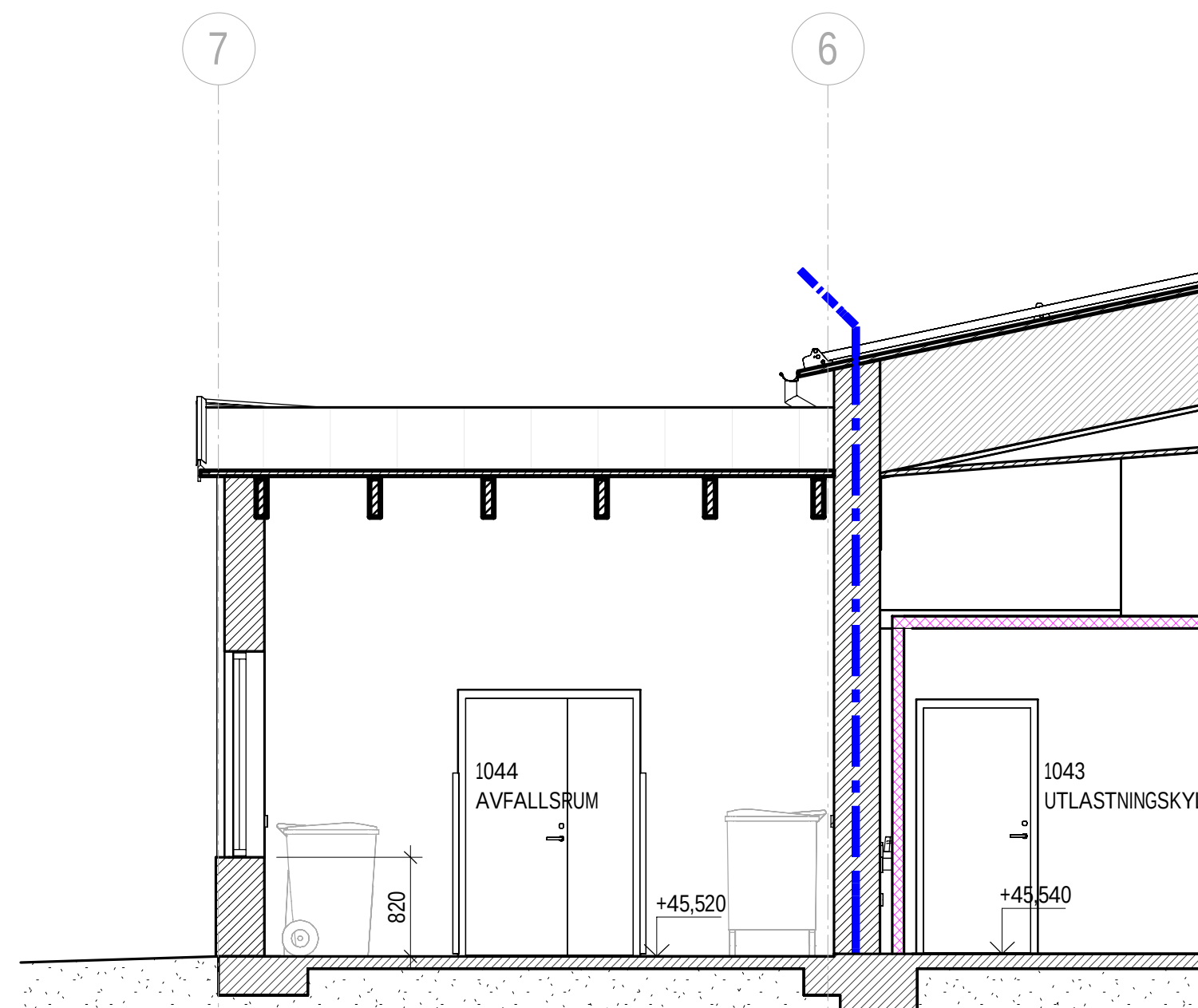
SEKTION C 1 : 50
