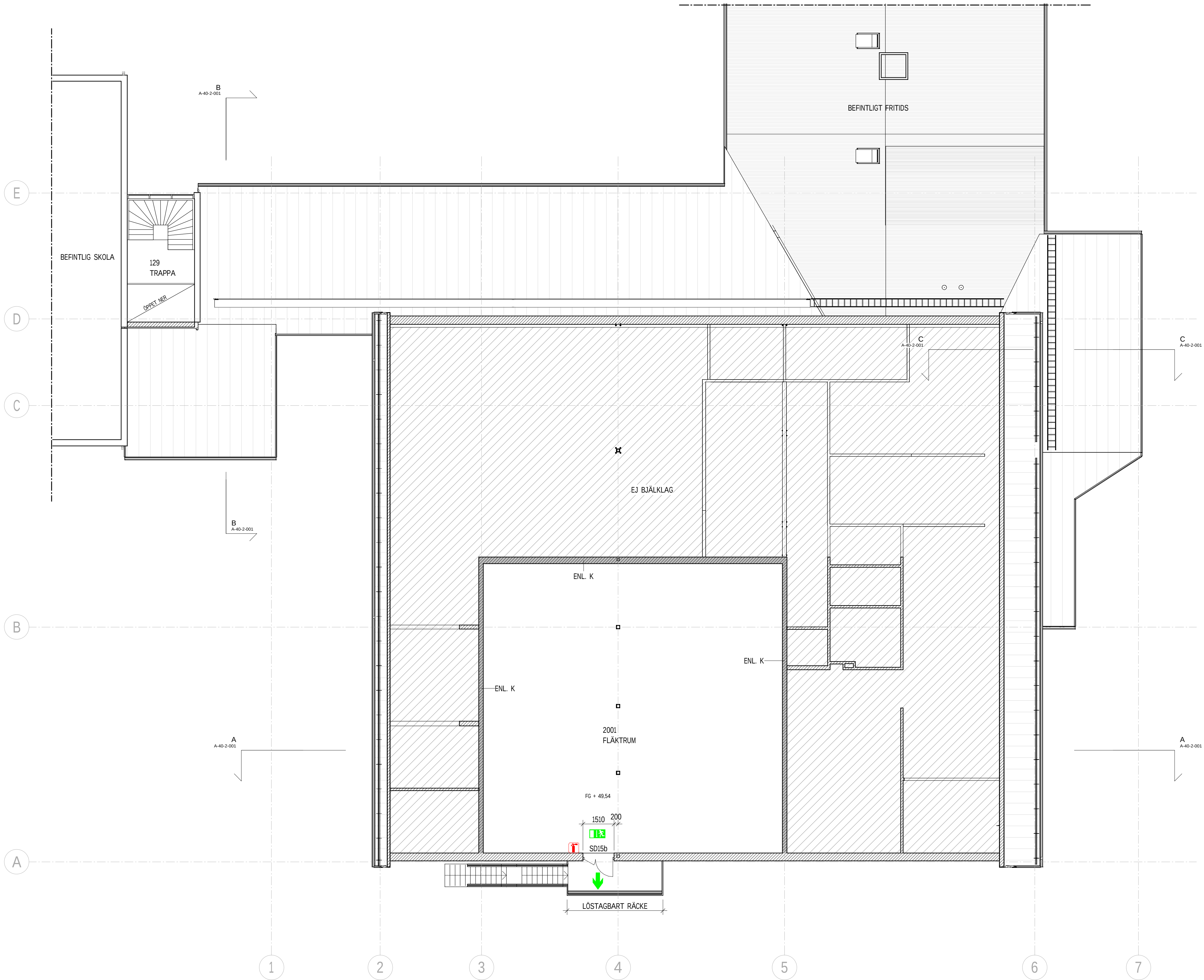
PLAN 2 1 : 100
