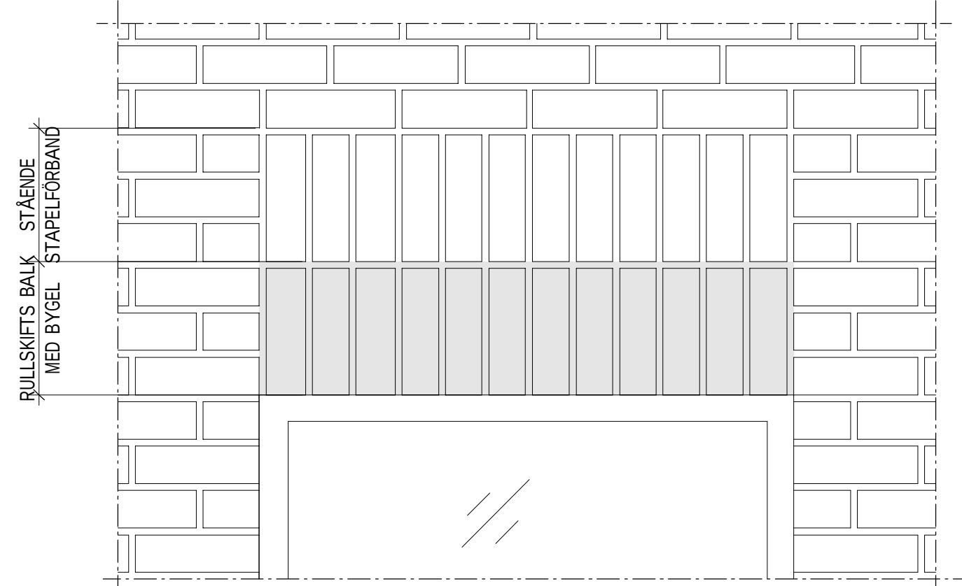
EV1 PRINCIP ELEVATION 1:10 RULLSKIFTS BALK - MED BYGEL
