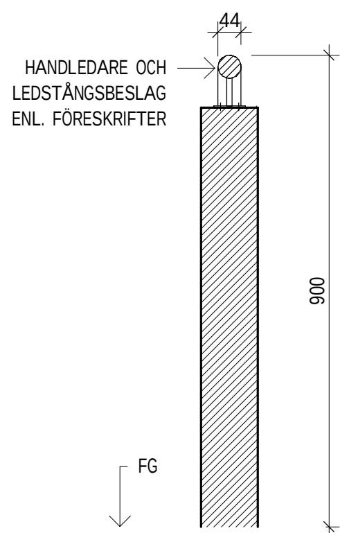
PRINCIPSEKTION HANDELDARE H2 1 : 10
