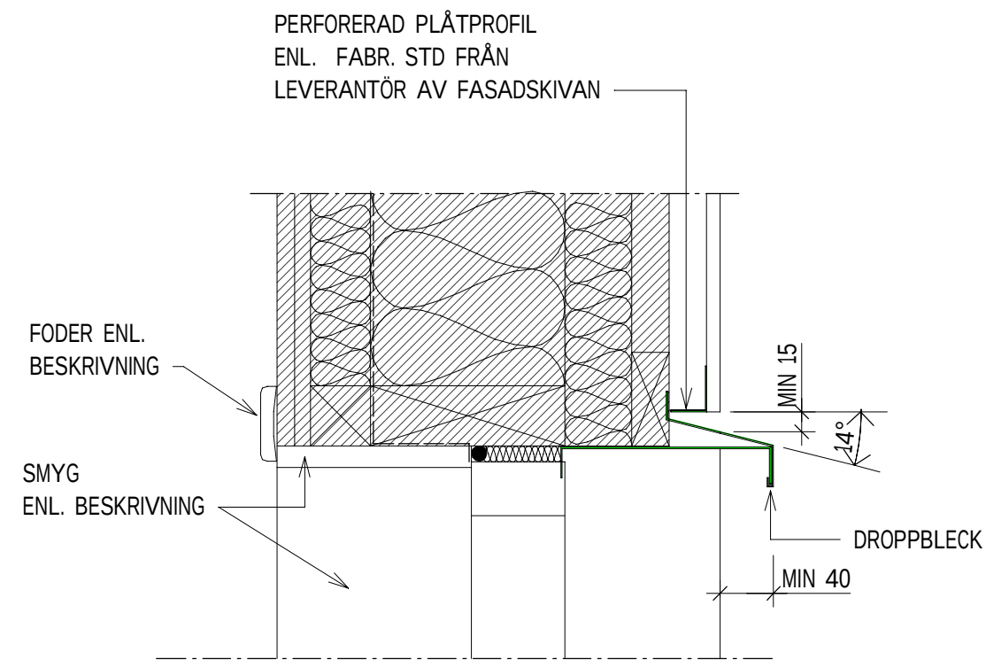
VD17 PRINCIPDETALJ 1:5 FÖNSTER SOPRUM
