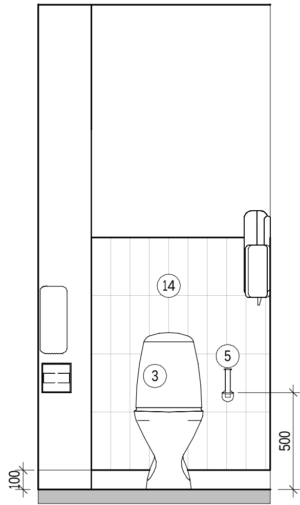
ELEVATION WC 1008 - A 1 : 20
