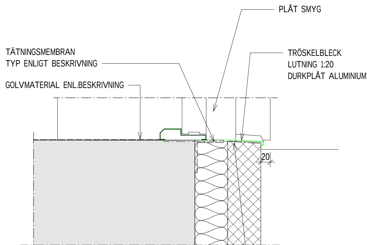
VD7 PRINCIPDETALJ 1:5 STÅLDÖRR
