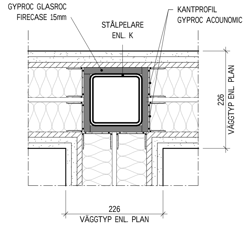
IK4 - STÅLPELARE I VÄGGKORSNING 1 : 5
