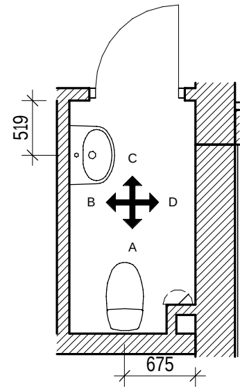
PLAN WC 1008 1 : 50
