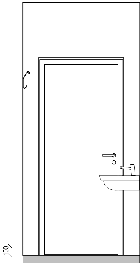
ELEVATION WC 1020 - B 1 : 20
