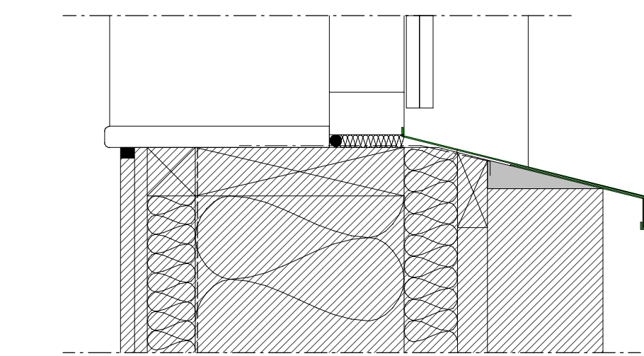
VD21 PRINCIPDETALJ 1:5 FÖNSTER MED VERTIKALMARKIS
