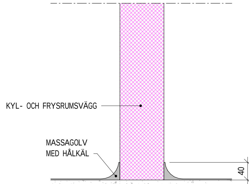
IVD12 - PRINCIPDETALJ MASSAGOLV MOT KYL-/FRYSRUMSVÄGG 1 : 5
