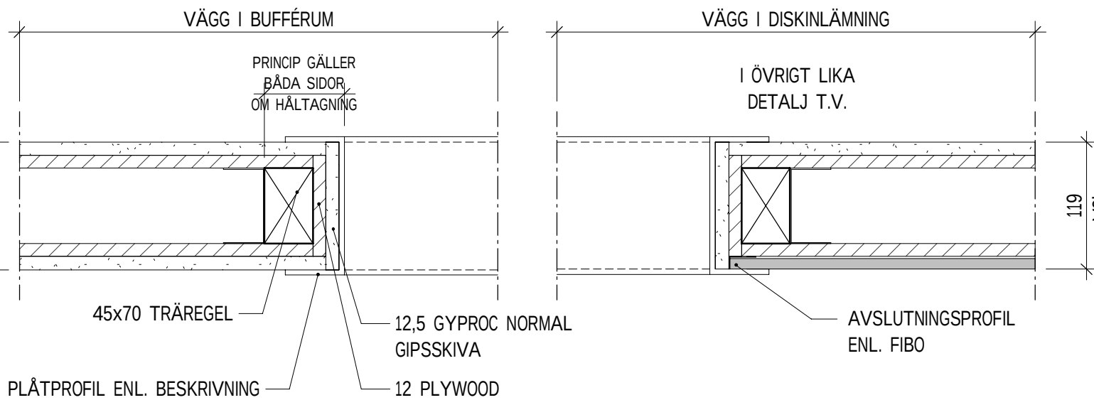
IVD07 - HÅLTAGNING VÄGG 1 : 5
