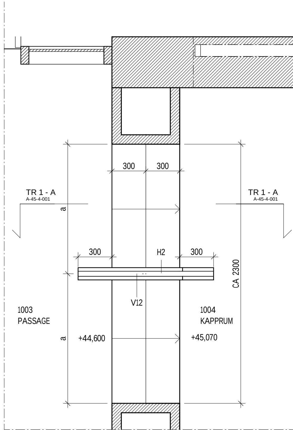
TRAPPA 1 - PLAN 1 : 20
