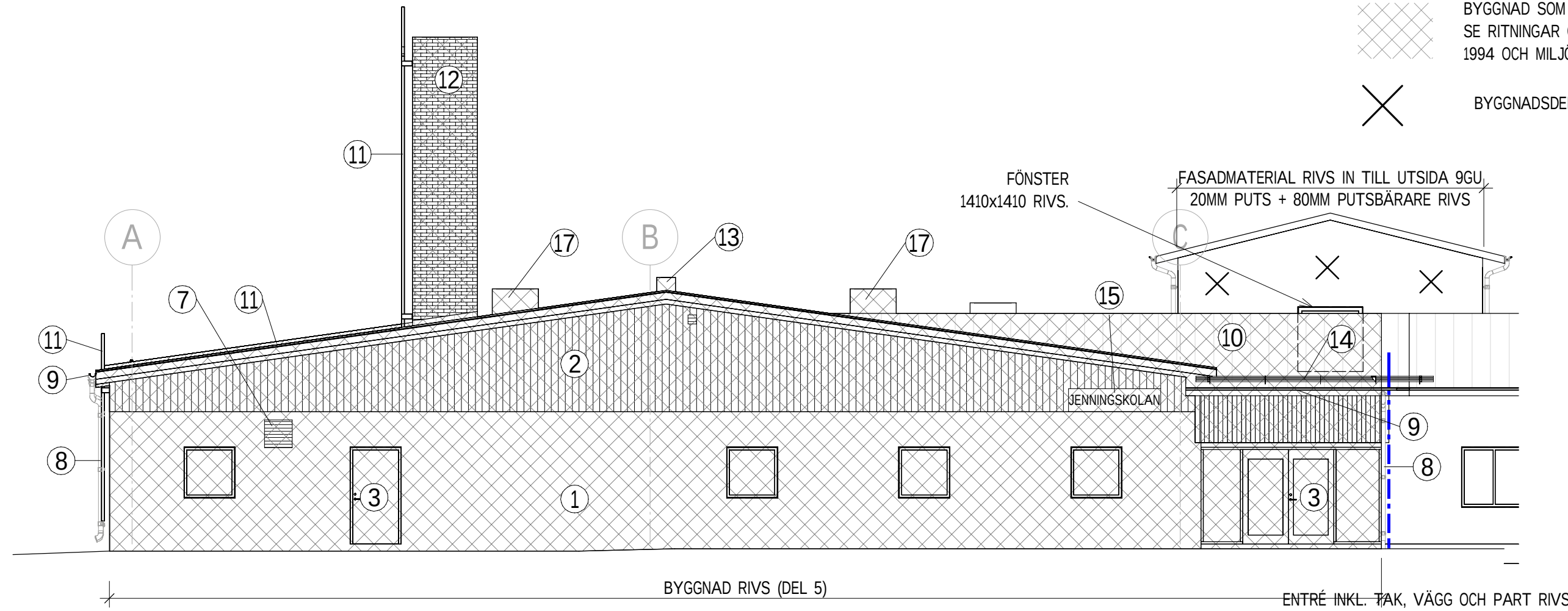
FASAD MOT NORDVÄST - RIVNING
