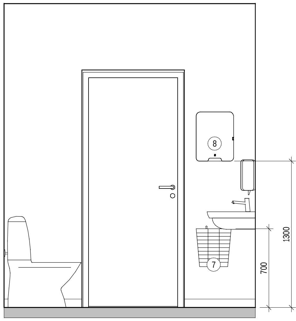
ELEVATION WC 1018 - B 1 : 20
