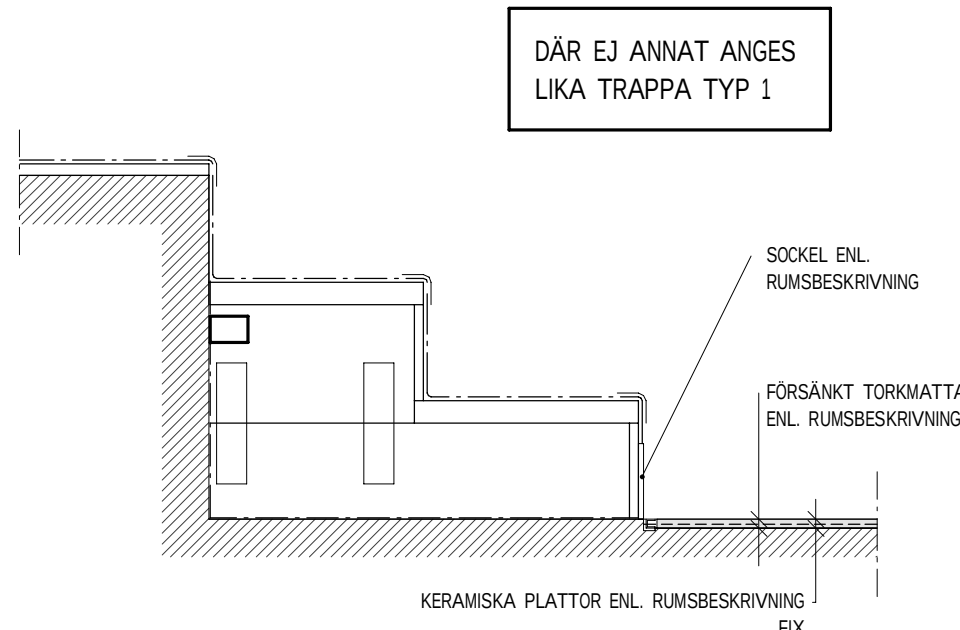
PRINCIPDETALJ TRAPPA TYP 2 1 : 10
