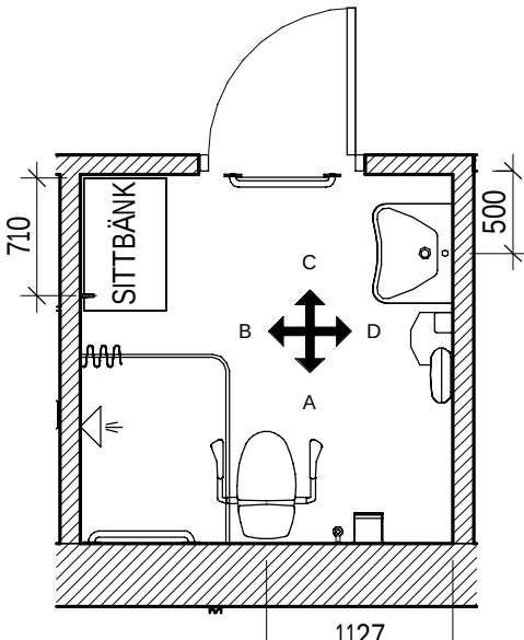
PLAN RWC/D 1016 1 : 50
