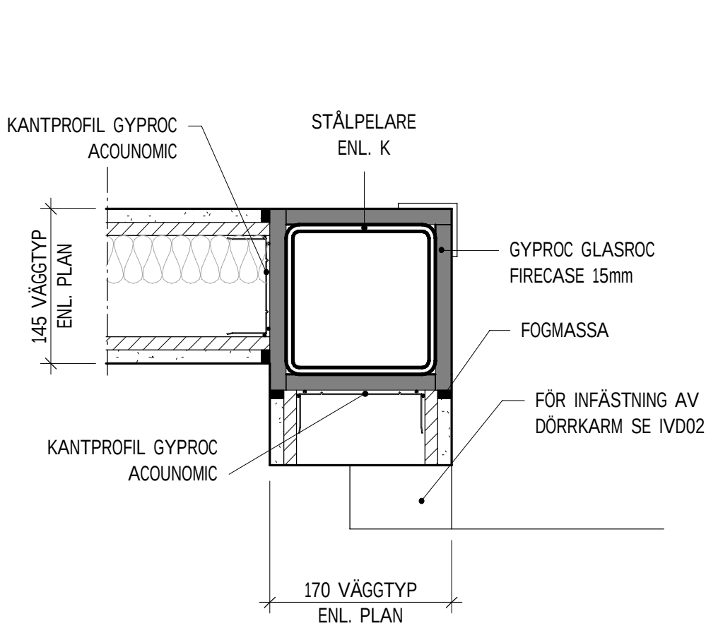
IK5 - STÅLPELARE I INNERVÄGGSHÖRN 1 : 5
