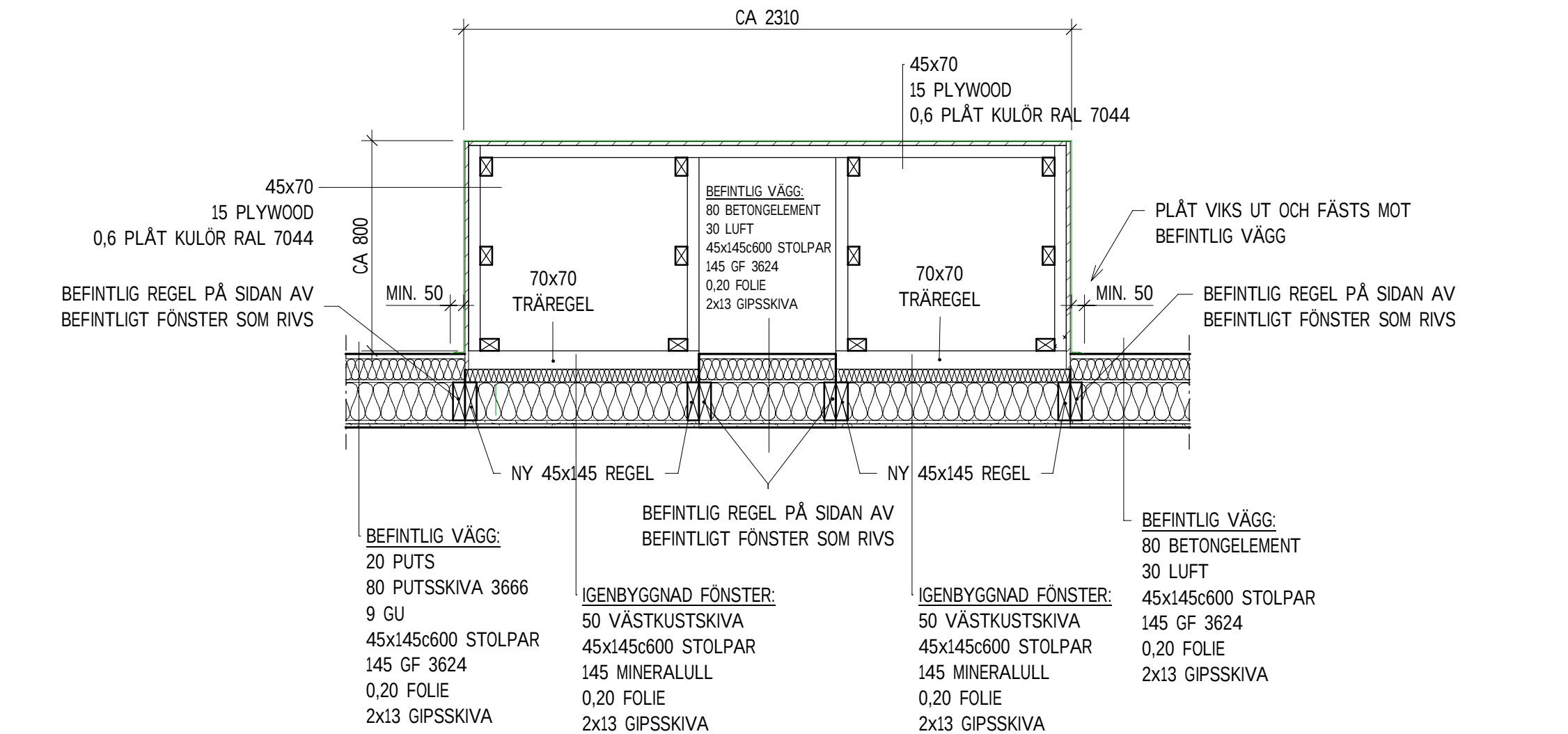
IGENBYGGNAD MOT UC, PLAN 1:20
