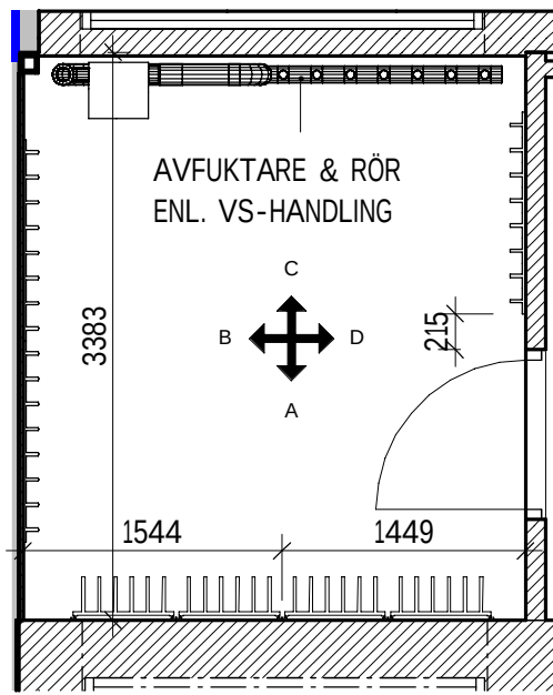
PLAN TORKRUM 1002 1 : 50
